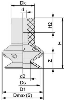
Tasarım verileri FGA 8 SI-HD-65 N063
