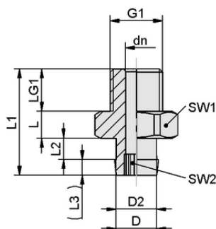
Données de construction SA-NIP N016 G1/8-AG DN350
