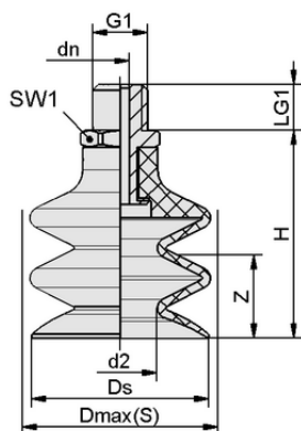
Dati di costruzione FSG 25 SI-MD-55 G1/8-AG
