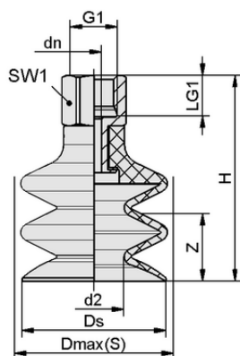
デザインデータ FSG 18 SI-MD-55 G1/8-IG
