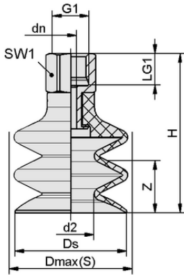
Tasarım verileri FSG 18 SI-MD-55 G1/8-IG
