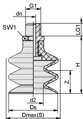
Конструктивные данные FSG 14 SI-MD-55 M5-AG
