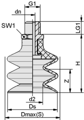
Datos de diseño FSG 14 SI-MD-55 M5-AG
