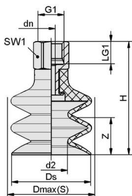
デザインデータ FSG 14 SI-MD-55 G1/8-IG
