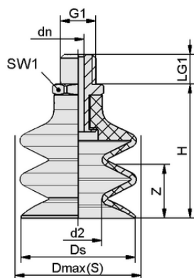
デザインデータ FSG 12 SI-MD-55 M5-AG
