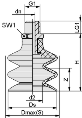
Tasarım verileri FSG 12 SI-MD-55 M5-AG
