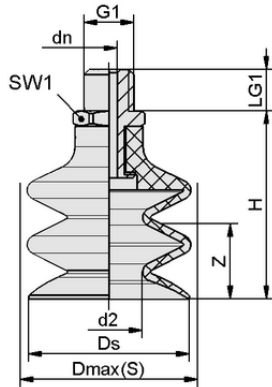
Tasarım verileri FSG 12 SI-MD-55 G1/8-AG
