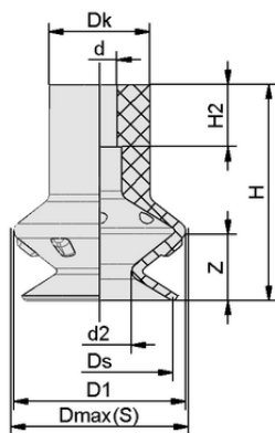
Datos de diseño FGA 8 SI-40 N063
