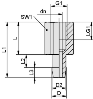
Tasarım verileri SA-NIP N062 G1/8-IG DN350
