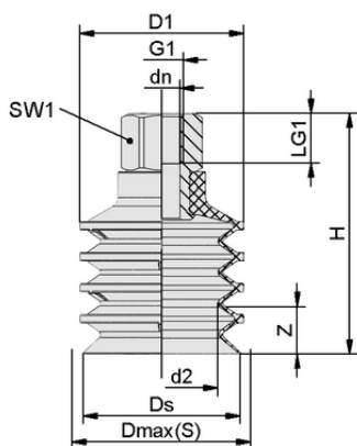
Dati di costruzione FSGC 40 NBR-55 G3/8-IG
