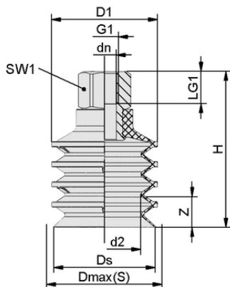
Dati di costruzione FSGC 40 NBR-55 G1/4-IG
