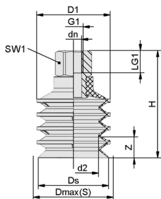
デザインデータ FSGC 50 NBR-55 G1/4-IG
