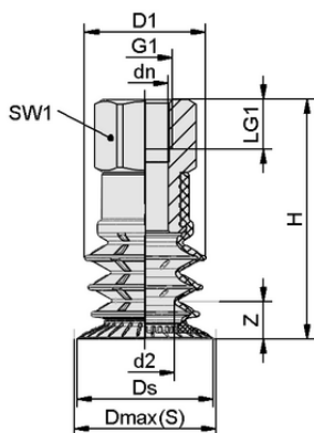
Datos de diseño PSPF 43 SI-30/55 G1/8-IG
