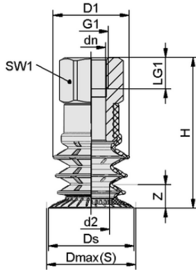
Tasarım verileri PSPF 33 SI-30/55 G1/4-IG
