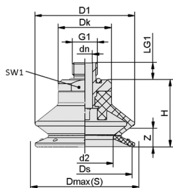
デザインデータ SDC1 60 PU 30/60 G3/8-AG
