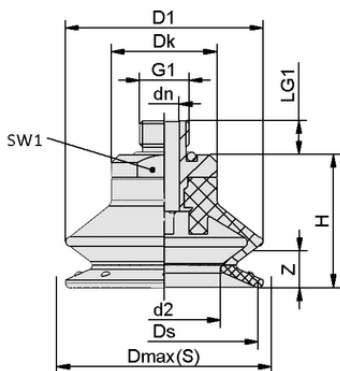
Données de construction SDC1 40 PU 30/60 G1/4-AG
