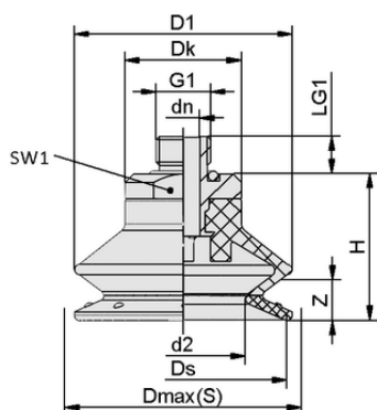
Dati di costruzione SDC1 20 PU 30/60 G1/8-AG
