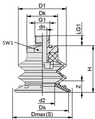
Dati di costruzione SDC2 50 PU 30/60 G3/8-AG
