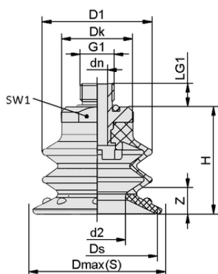
デザインデータ SDC2 40 PU 30/60 G1/4-AG
