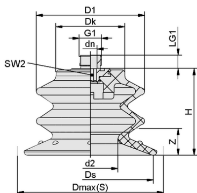
デザインデータ SDC2 75 PU 30/60 G3/8-AG
