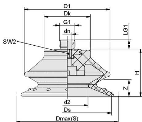
デザインデータ SDC1 100 PU 30/60 G3/8-AG
