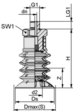
Datos de diseño SPB4f 50 SI-55 NPT3/8-AG
