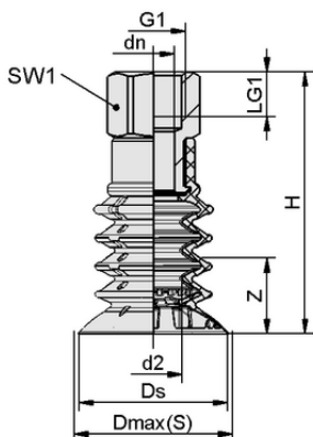
Datos de diseño SPB4f 40 SI-55 NPT3/8-IG
