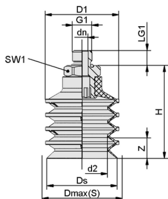
デザインデータ FSGC 50 NBR-55 G1/4-AG
