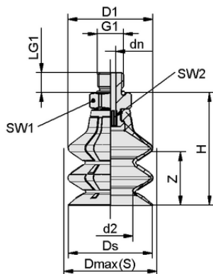
Datos de diseño SPB2 25 ED-65 NPT1/8-AG
