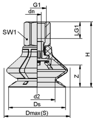
Datos de diseño SPB1 40 ED-65 NPT1/4-IG
