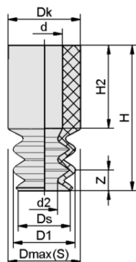
Конструктивные данные FG 52 SI-MD-55 N018
