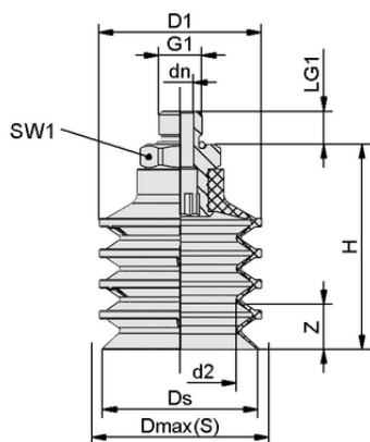
Datos de diseño FSGC 40 NBR-55 G1/4-AG
