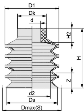
Конструктивные данные FGC 40 NBR-55 SC080
