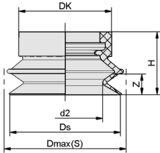
Tasarım verileri BCG 50 SI-HD-65 SC095
