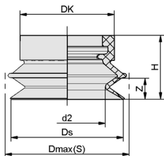
Конструктивные данные BCG 40 SI-HD-65 SC095
