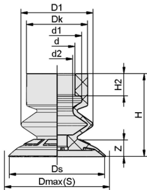
Dati di costruzione SFB1 20 NBR-ESD-55 SC040
