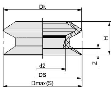
Конструктивные данные FLSA 40 SI-MD-55
