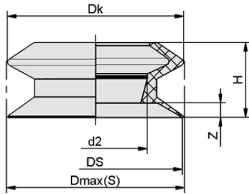
Tasarım verileri FLSA 20 SI-MD-55
