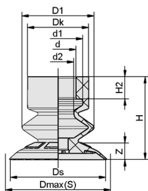
Конструктивные данные SFB1 10 NBR-ESD-55 SC030
