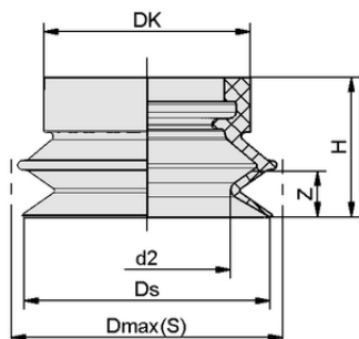
デザインデータ BCG 40 NBR-ESD-55 SC095
