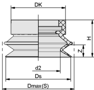
Konstruktionsdaten BCG 50 SI-MD-55 SC095
