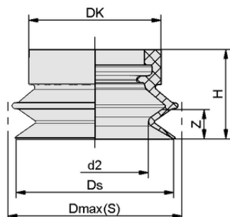
Конструктивные данные BCG 20 SI-MD-55 SC085
