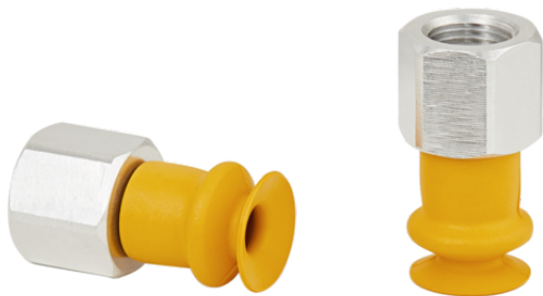
FSGA 16 NBR-ESD-55 G1/8-IG
