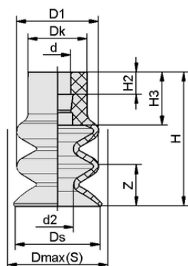
デザインデータ FG 25 NBR-ESD-55 N062
