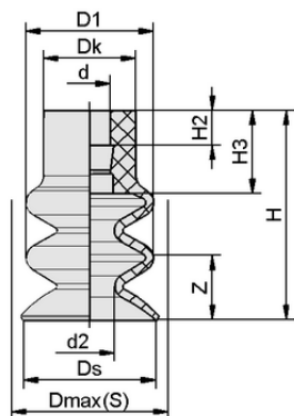
デザインデータ FG 18 NBR-ESD-55 N062
