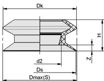
Konstruktionsdaten FLSA 50 NBR-ESD-55
