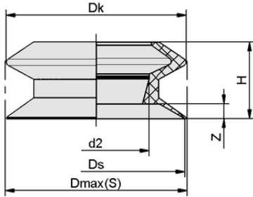
Tasarım verileri FLSA 50 NBR-ESD-55
