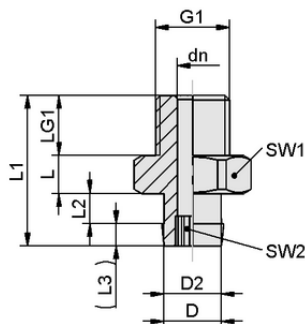
Dati di costruzione SA-NIP N016 M5-AG DN250
