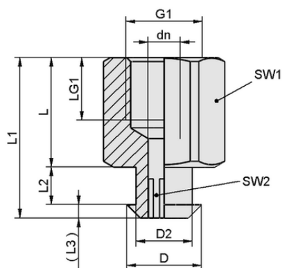
Datos de diseño SC 050 G1/4-IG SW410
