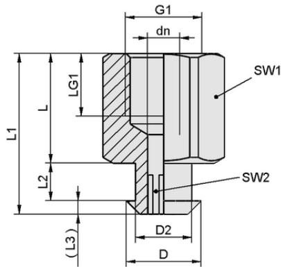
Tasarım verileri SC 050 G1/4-IG SW410
